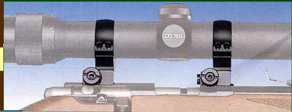
Aufschub-Montage
